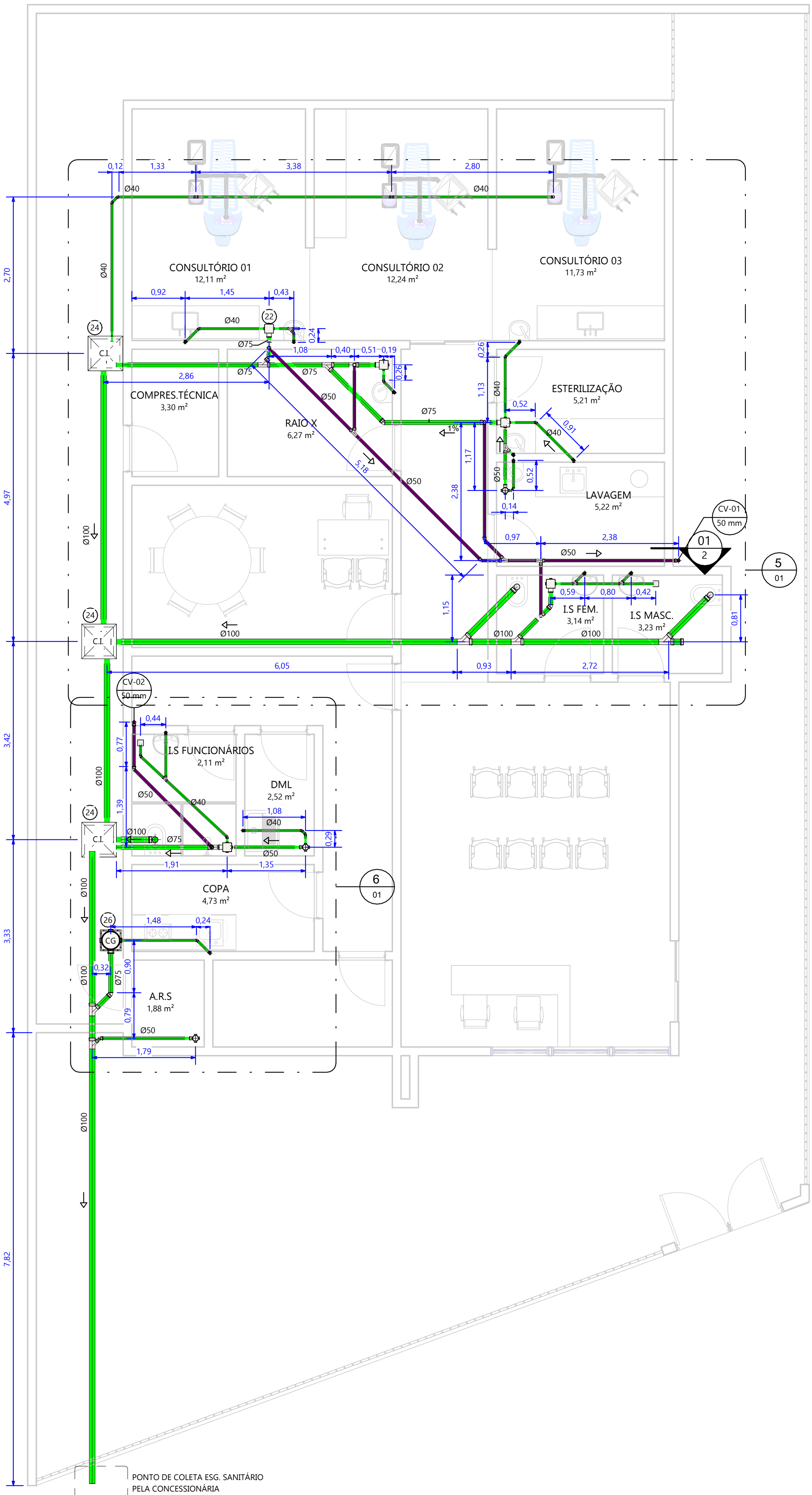
1 TÉRREO ESC: 1 : 50
