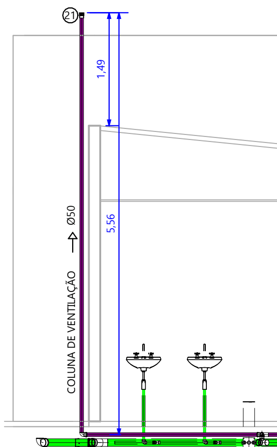
2 COLUNA DE VENTILAÇÃO ESC: 1 : 50
