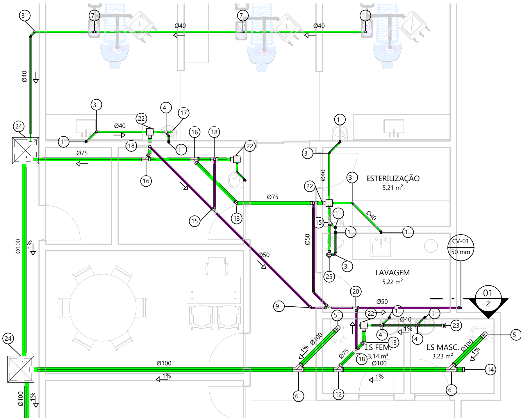
5 TÉRREO - Ampliação 02 ESC: 1 : 50
