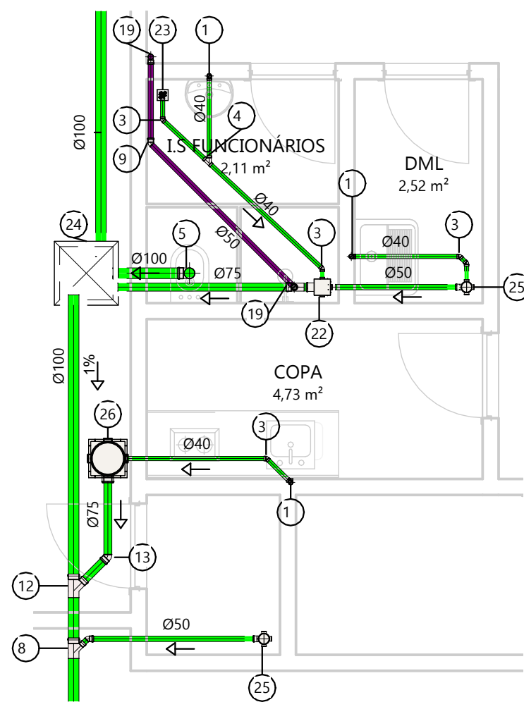
6 TÉRREO - Ampliação 01 ESC: 1 : 50
