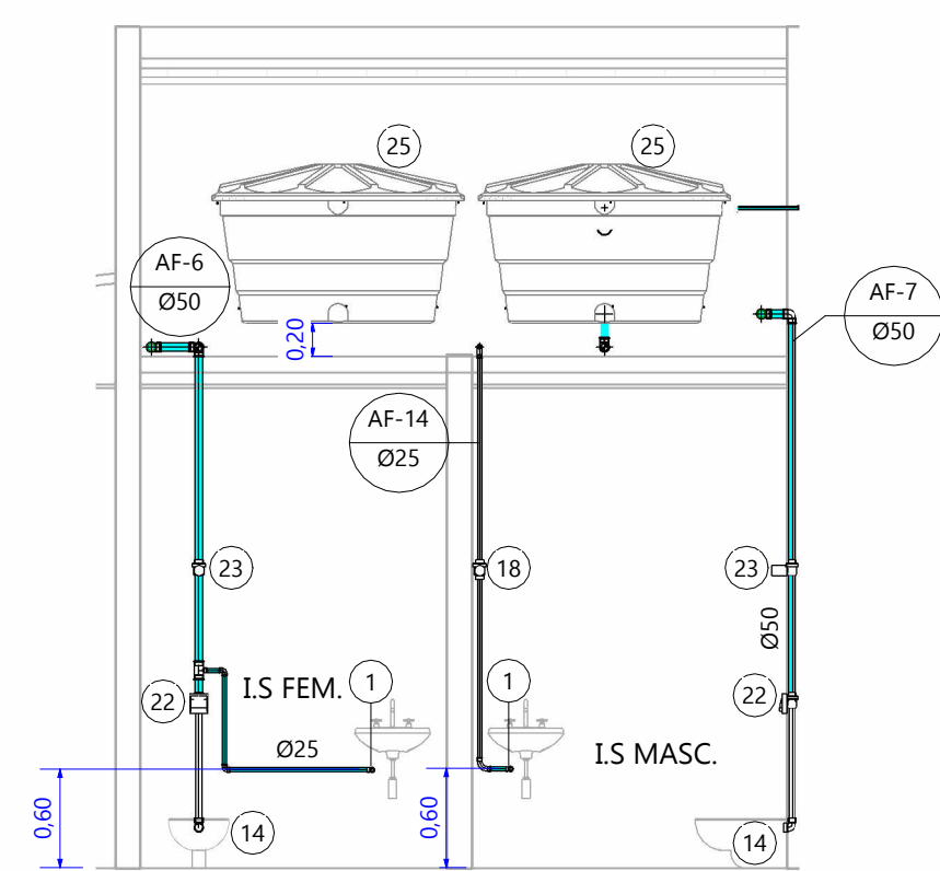
6 DET-06-ELEVAÇÃO-06 ESC: 1 : 50
