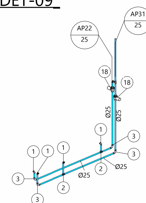
13 ISOMÉTRICO-DET-09 Sem Escala
