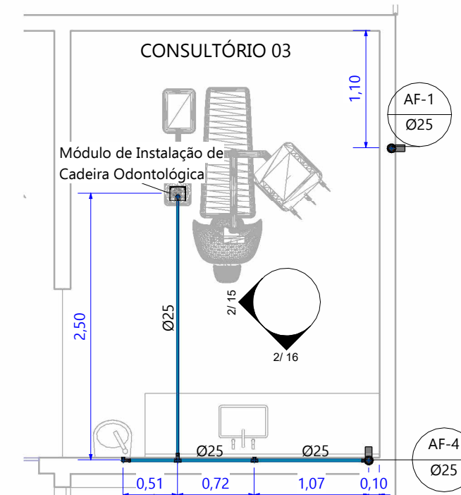
12 PLANTA - DET-06 ESC: 1 : 50
