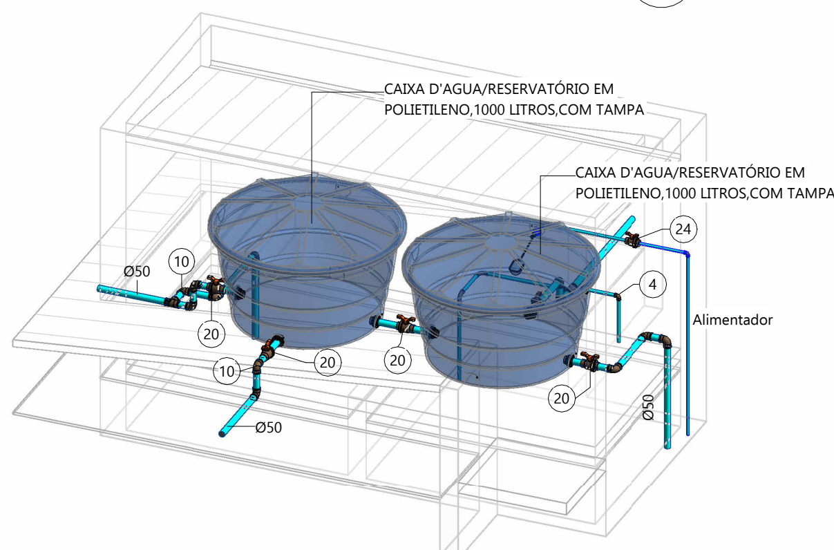
2 ISOMÉTRICO Sem Escala
