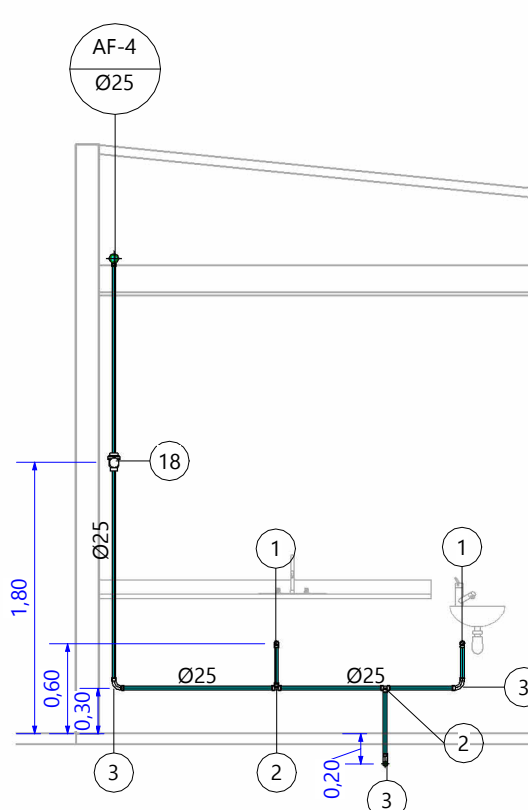
16 DET-07-ELEVAÇÃO-07 ESC: 1 : 50
