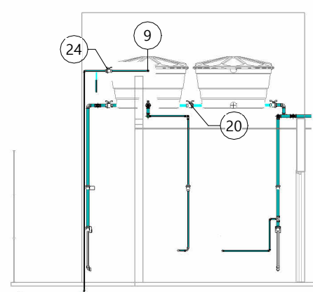
6 RESERVATÓRIO ESC: 1 : 100
