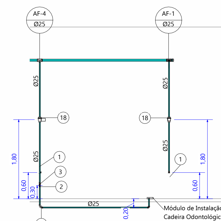
15 DET-08-ELEVAÇÃO-08 ESC: 1 : 50
