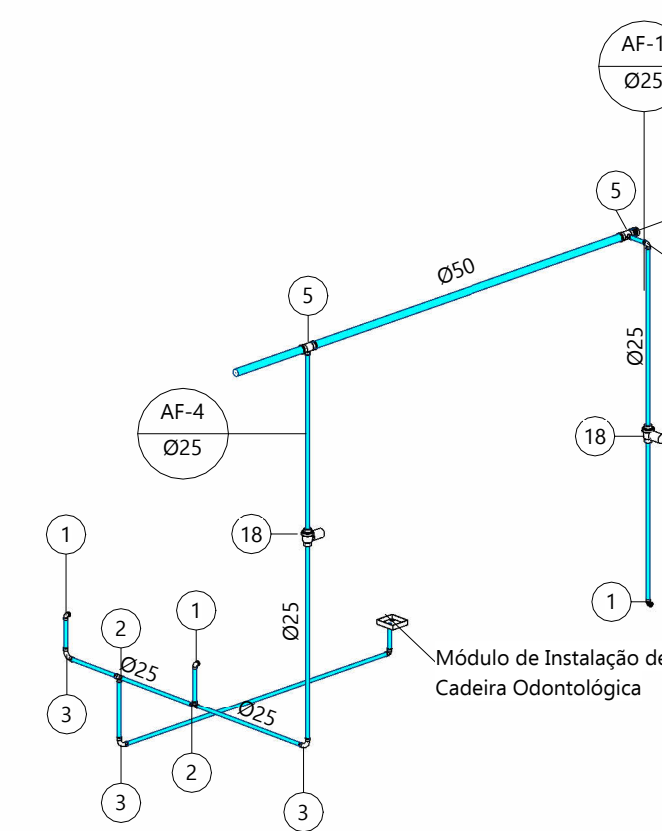
13 ISOMÉTRICO-DET-09 Sem Escala
