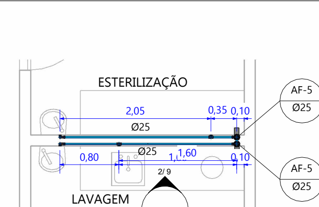
8 PLANTA - DET-08 ESC: 1 : 50
