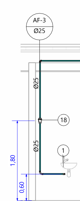
17 DET-04-ELEVAÇÃO-04 FSC: 1:50
