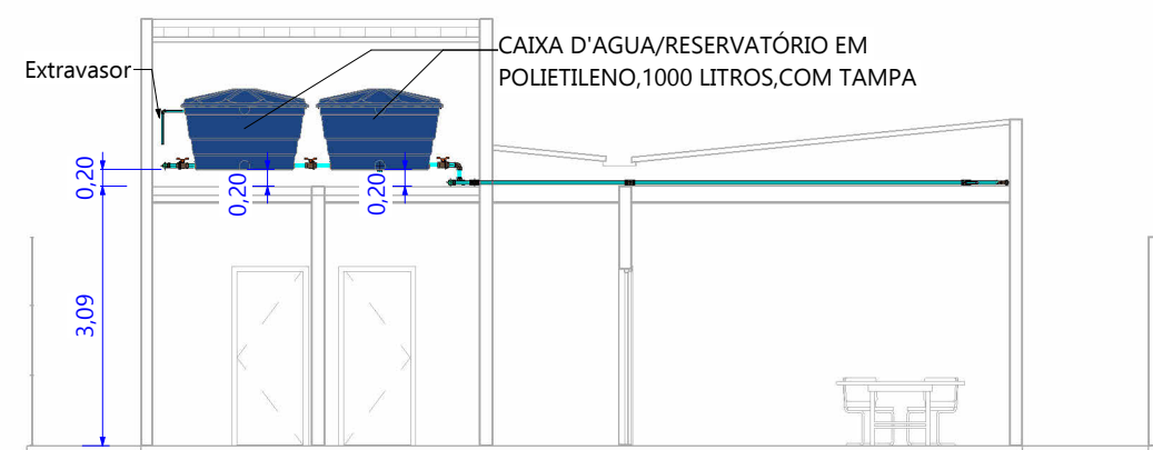
3 CORTE TRANSVERSAL ESC: 1 : 100
