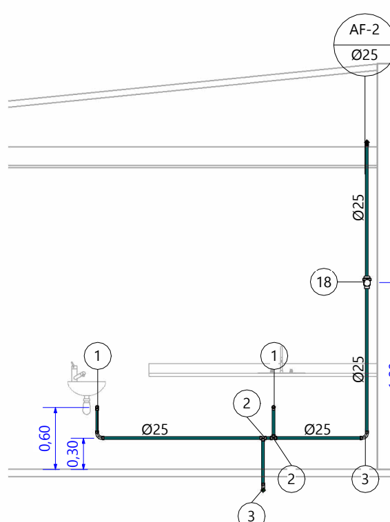
19 DET-02 -ELEVAÇÃO-02 ESC: 1 : 50
