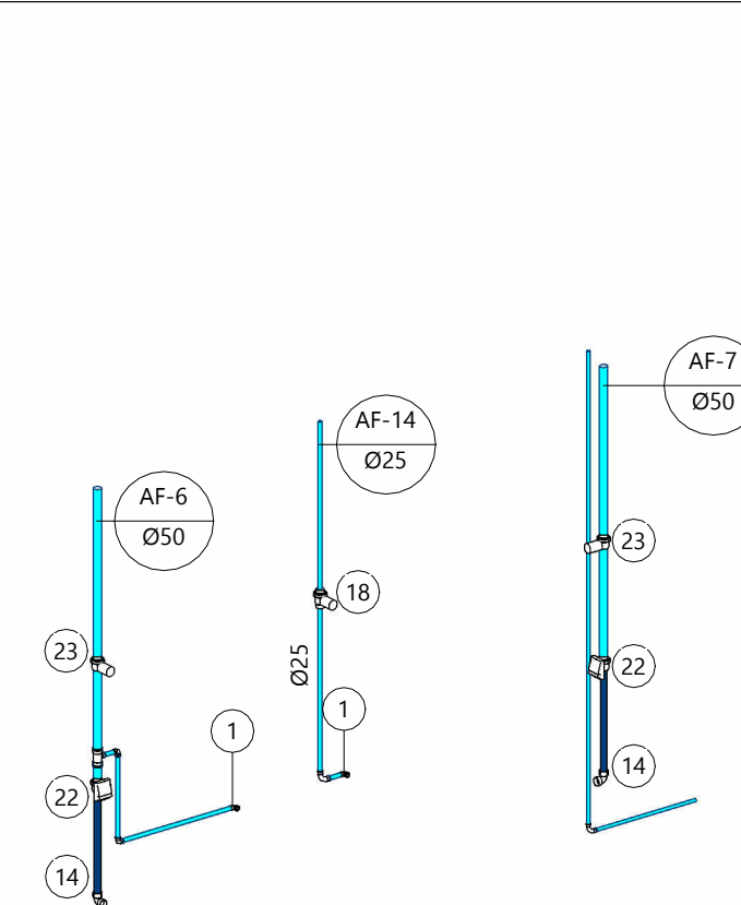
7 ISOMÉTRICO-DET-07 Sem Escala
