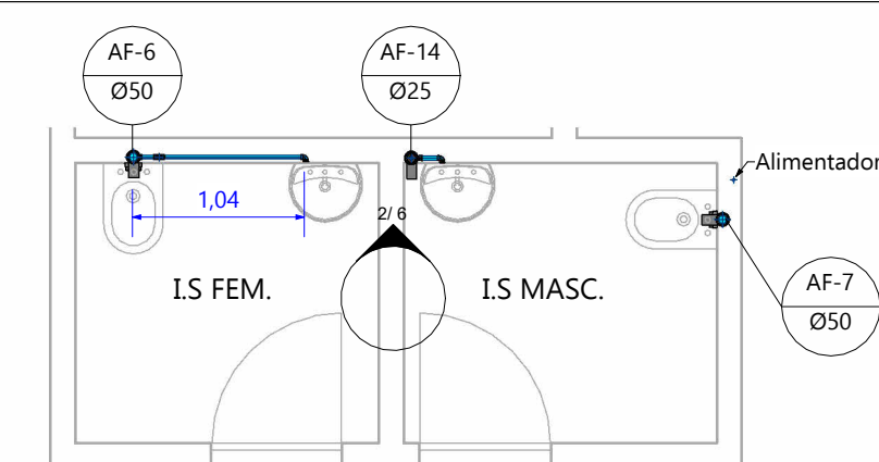
5 PLANTA - DET-05 ESC: 1:50
