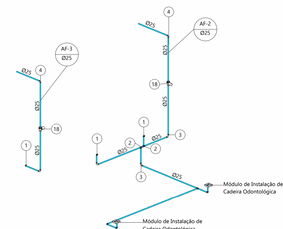
14 ISOMÉTRICO- DET-05 Sem Escala
