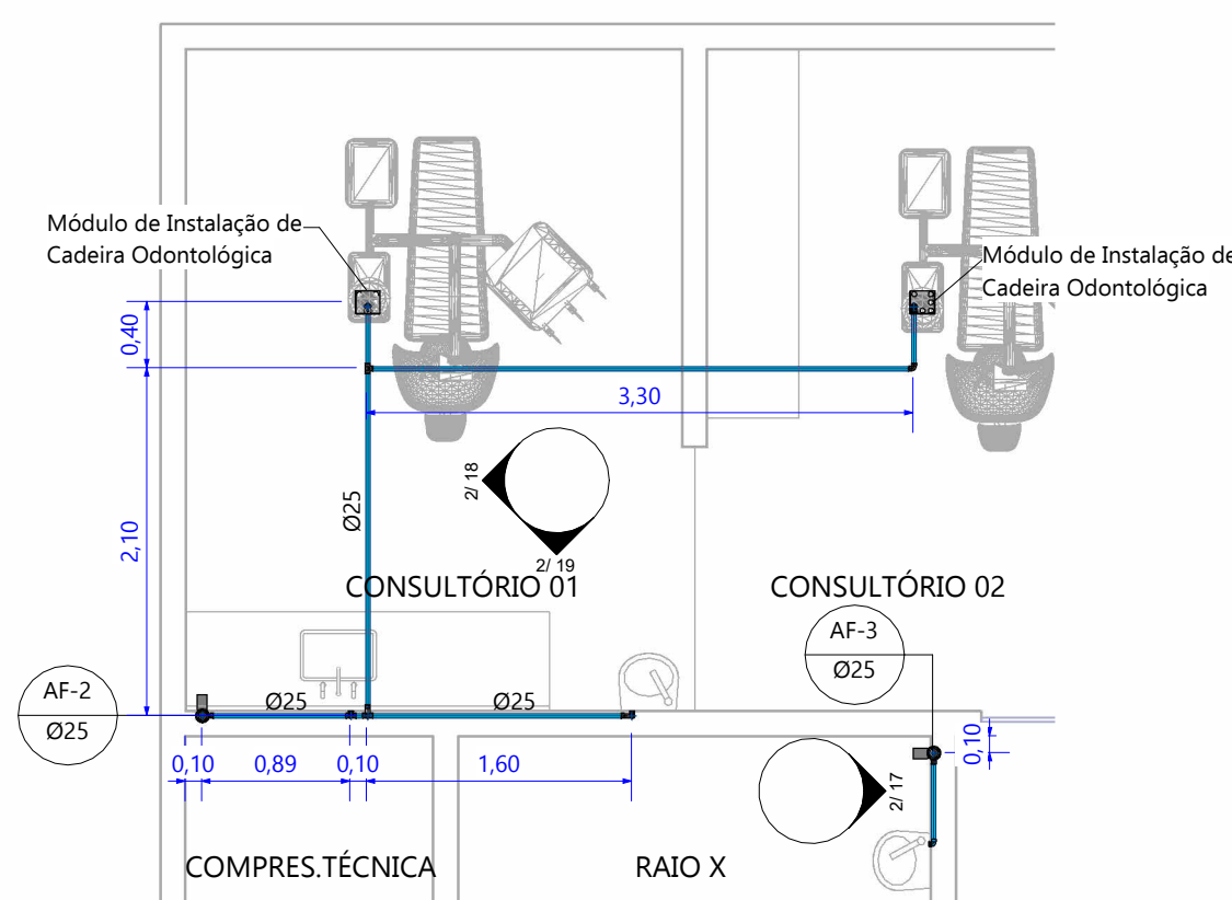
11 PLANTA - DET-01 ESC: 1 : 50
