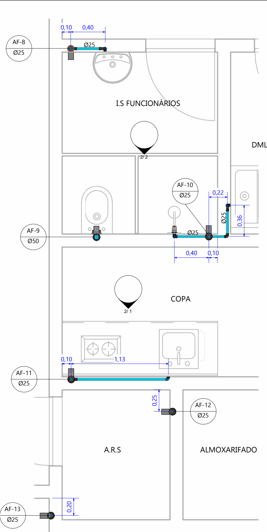
3 PLANTA - DET-03 ESC: 1:25
