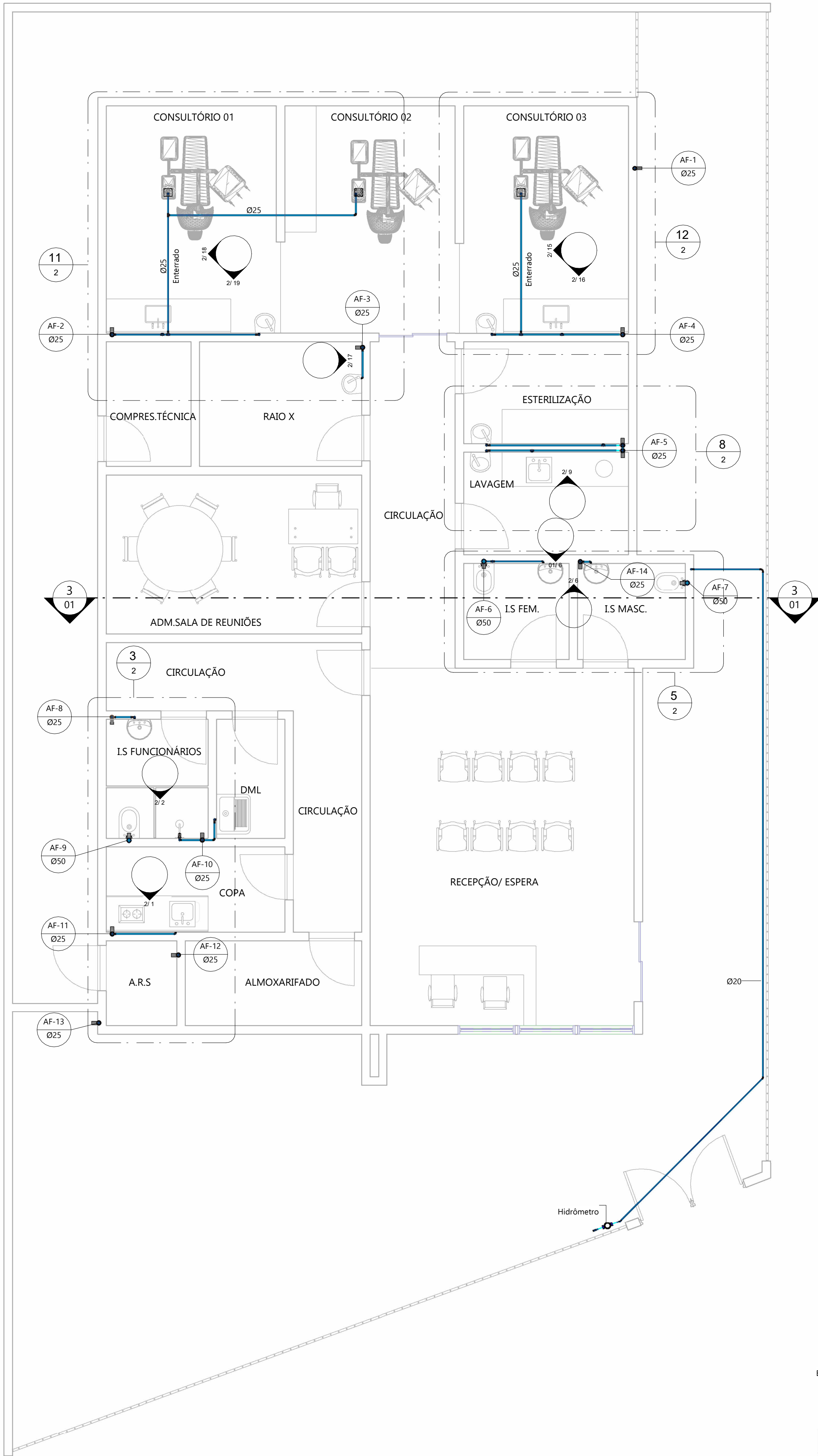
1 PLANTA ESC: 1 : 50
