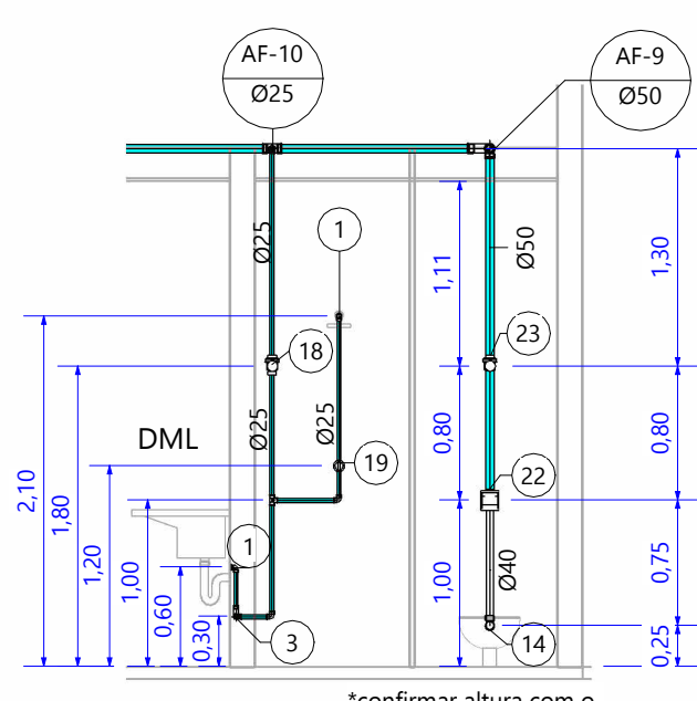
2 DET-02-ELEVAÇÃO-02 ESC: 1 : 50
