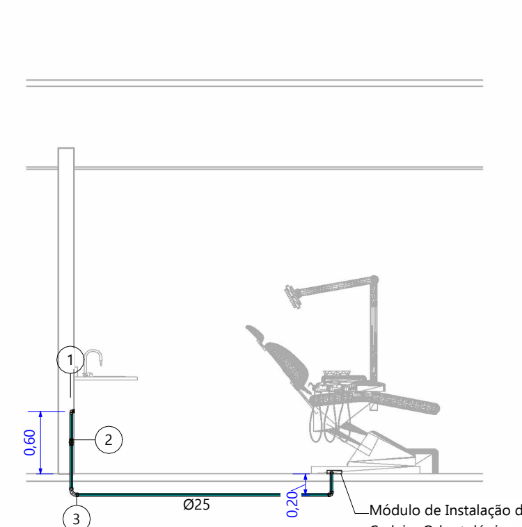
18 DET-03-ELEVAÇÃO-03 ESC: 1 : 50
