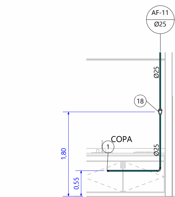
1 DET-01-ELEVAÇÃO-01 ESC: 1 : 50
