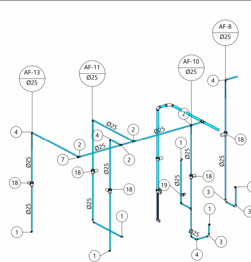
4 ISOMÉTRICO DET-04 Sem Escala
