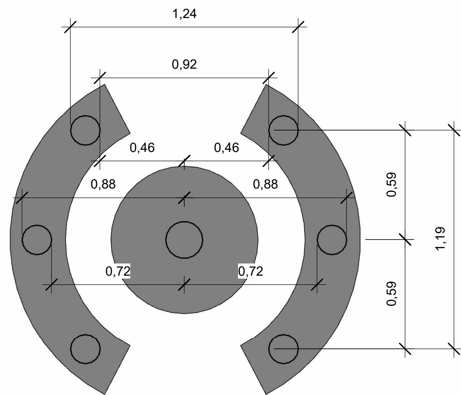
5 DETALHE 2 CONJUNTO MESA E BANCOS DE CONCRETO 1 : 20
