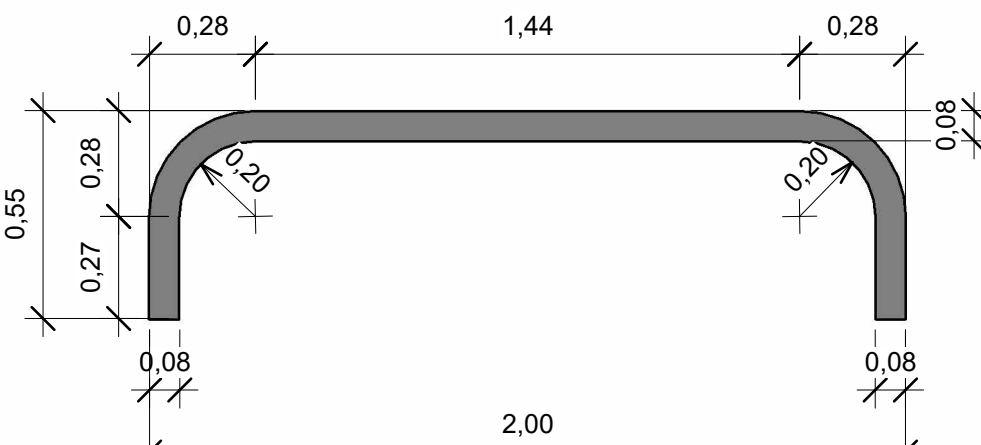
10 CORTE BANCO DE CONCRETO 1 : 20
