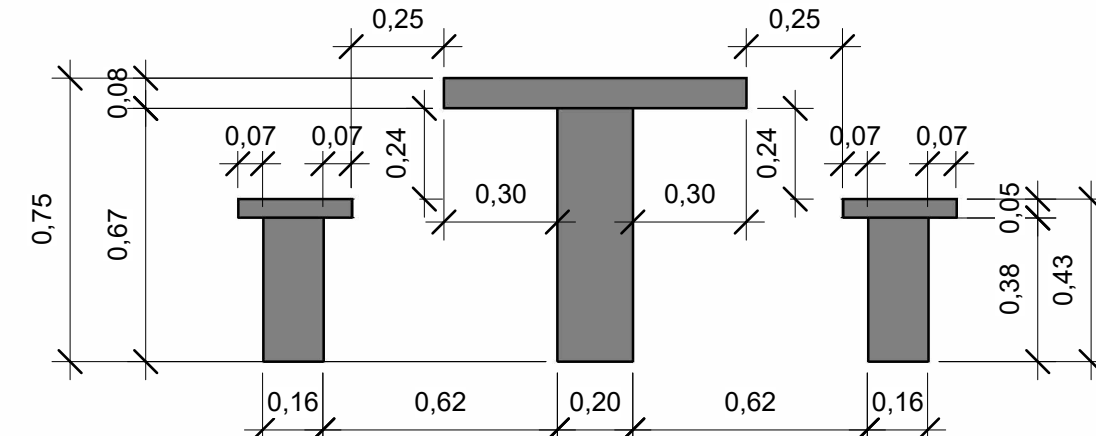
6 CORTE CONJUNTO MESA E BANCOS 1 : 20
