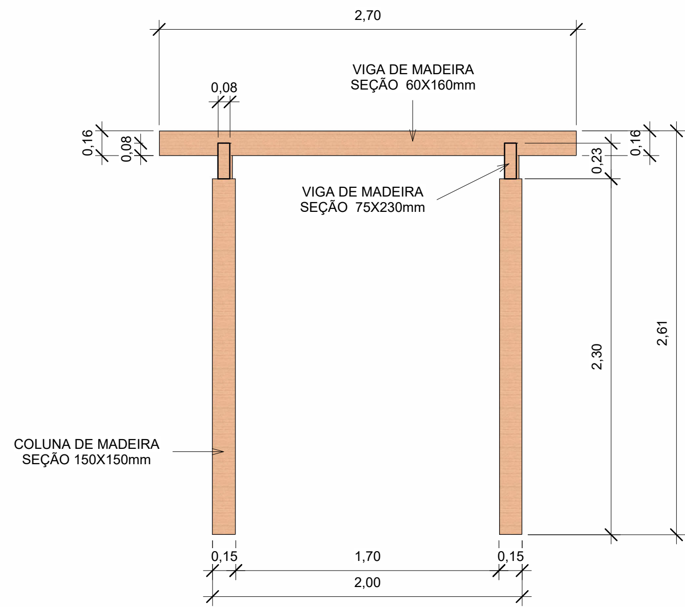
2 CORTE PERGOLADO 1 : 25
