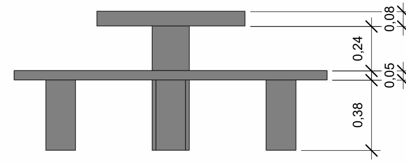
7 CORTE 2 CONJUNTO MESA E BANCOS 1 : 20
