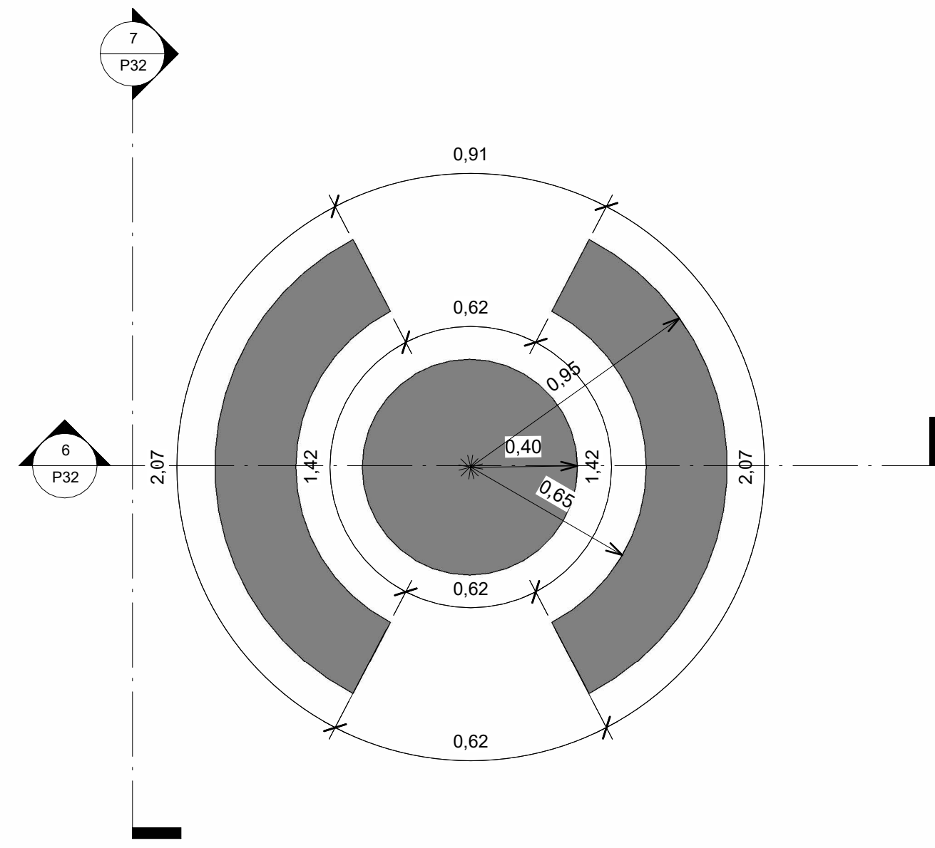
4 DETALHE CONJUNTO MESA E BANCOS DE CONCRETO 1 : 20
