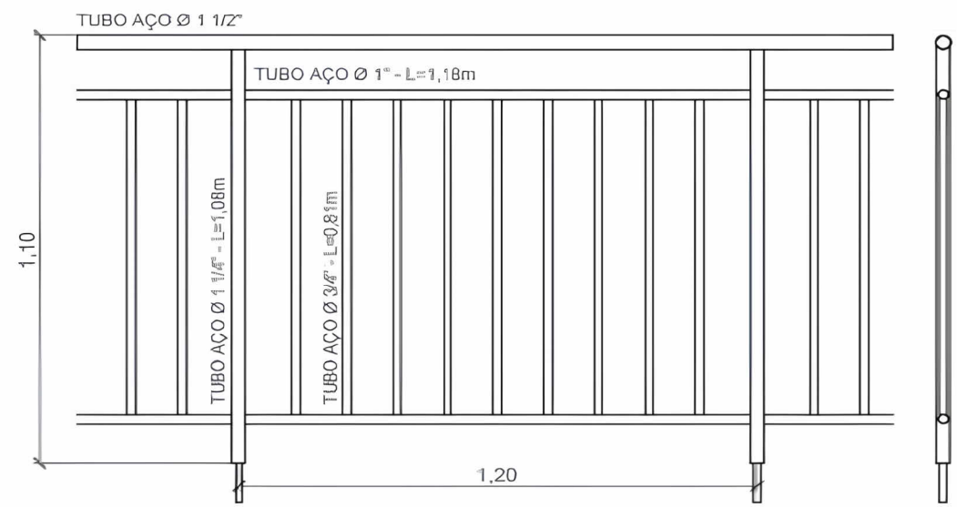
DETALHE GUARDA CORPO METÁLICO
