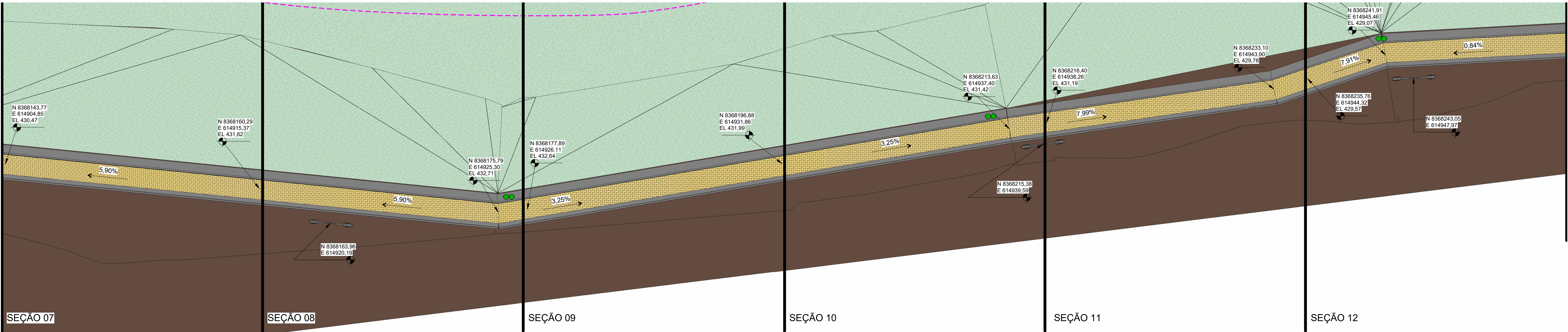
PAVIMENTAÇÃO INFERIOR - SEÇÃO 07 à 12
