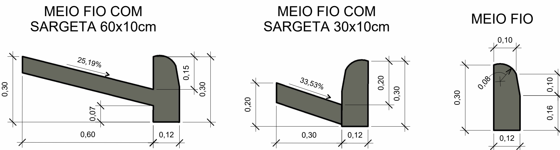
DETALHE GUIAS E SARJETAS
