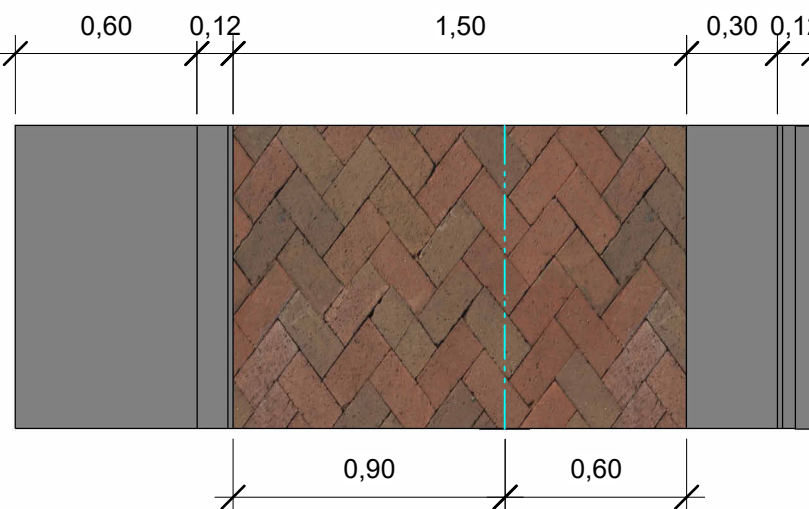
DETALHAMENTO PAVIMENTAÇÃO TIPO 1
