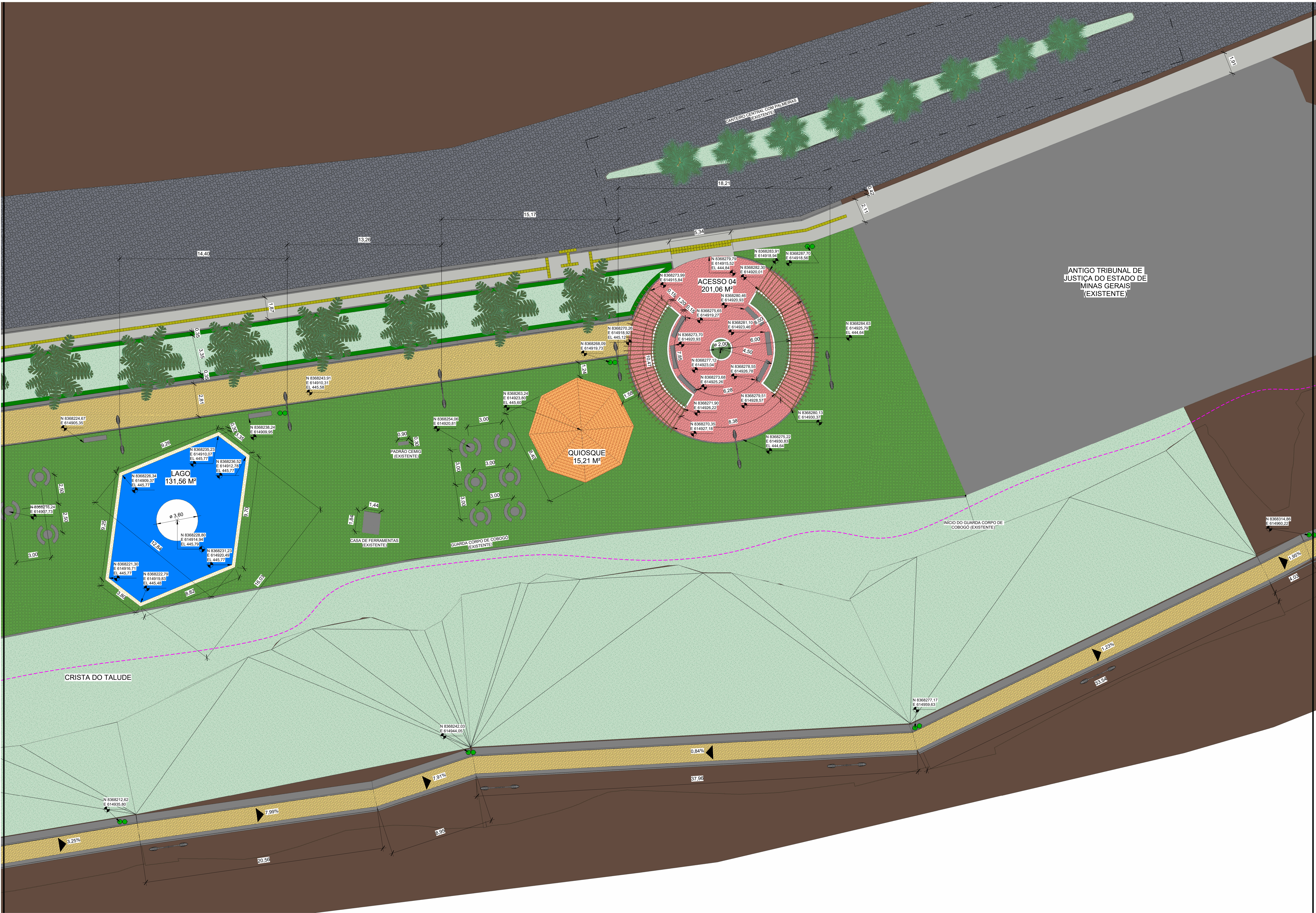
1 TRECHO 06 1 : 120
