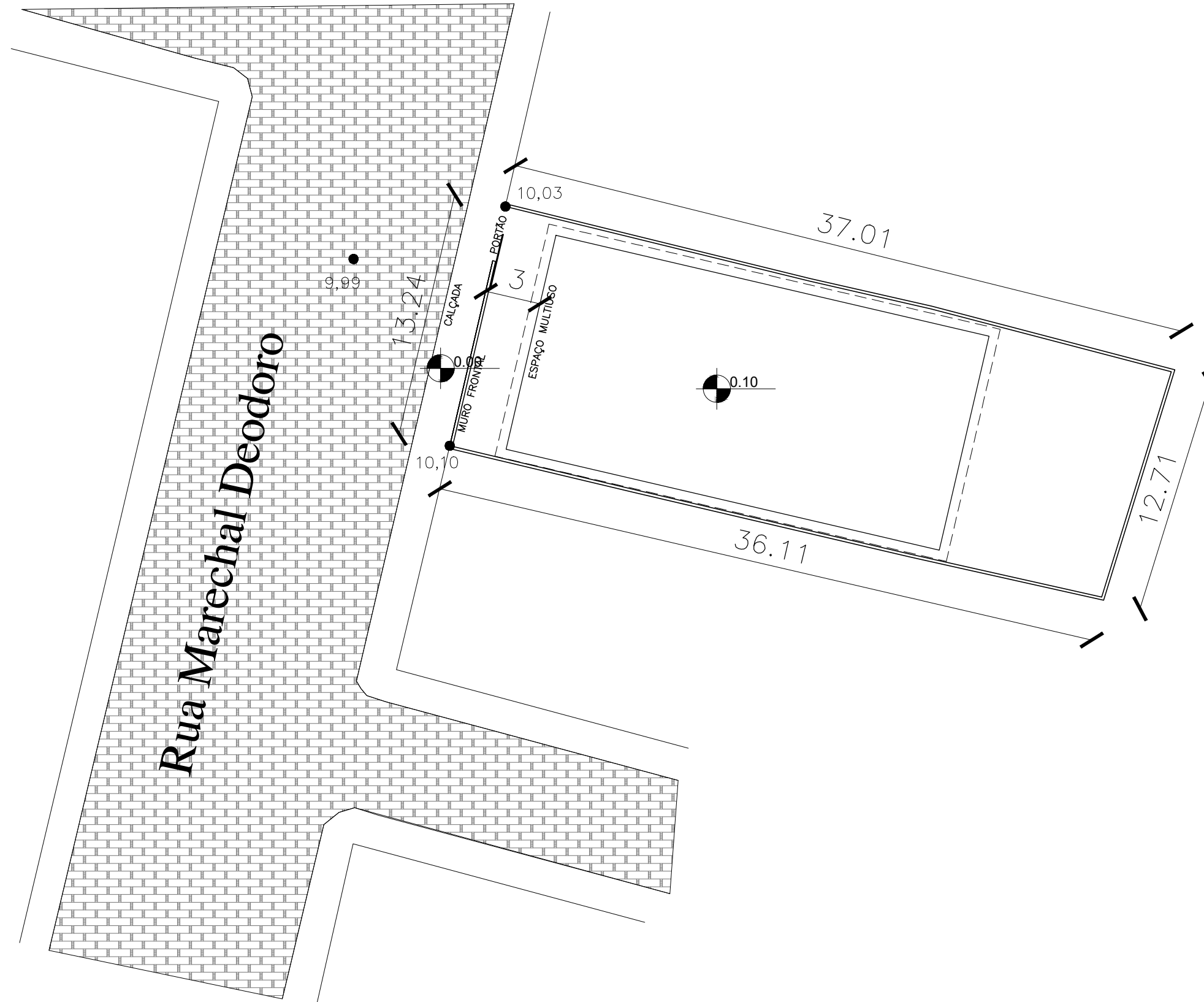
PLANTA DE LOCAÇÃO Escala 1/250
