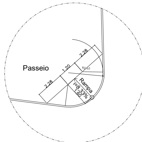
Detalhe rampa sem escala
